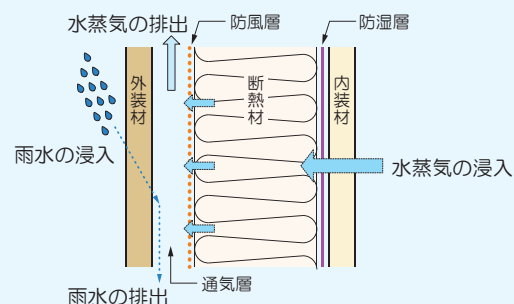
断熱壁体の構成
